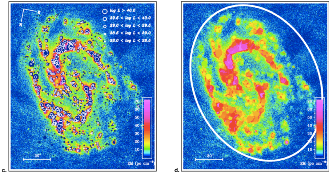
NGC 157
