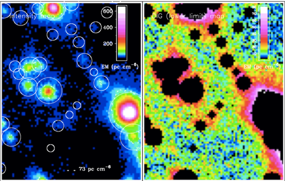
NGC 157
